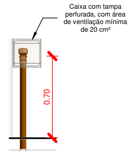
DETALHE - VÁLVULA DE ADMISSÃO DE AR 1 : 20
